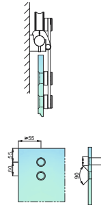
Aplicação Parede Vidro
