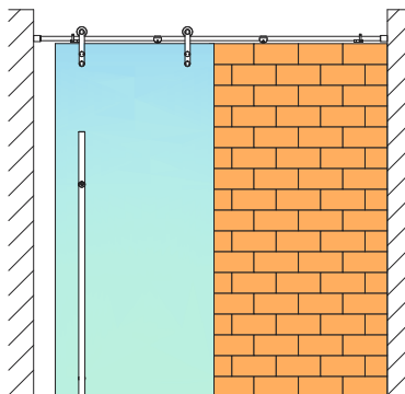
Aplicação Parede Vidro
