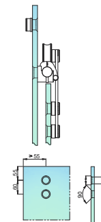
Aplicação Vidro Vidro
