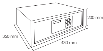
iSB-01 430x200x350mm
