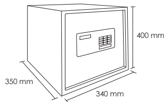
iSB-03 340x400x350mm
